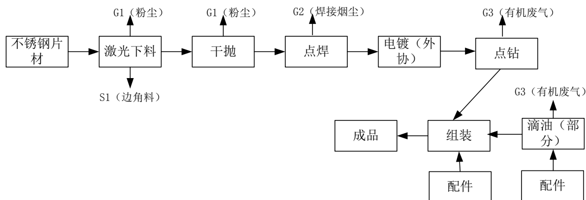
图 1-1 不锈钢饰品生产工艺流程图
