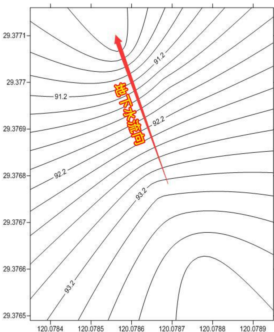
图 3.1.5-1 地下水流向等值线图
