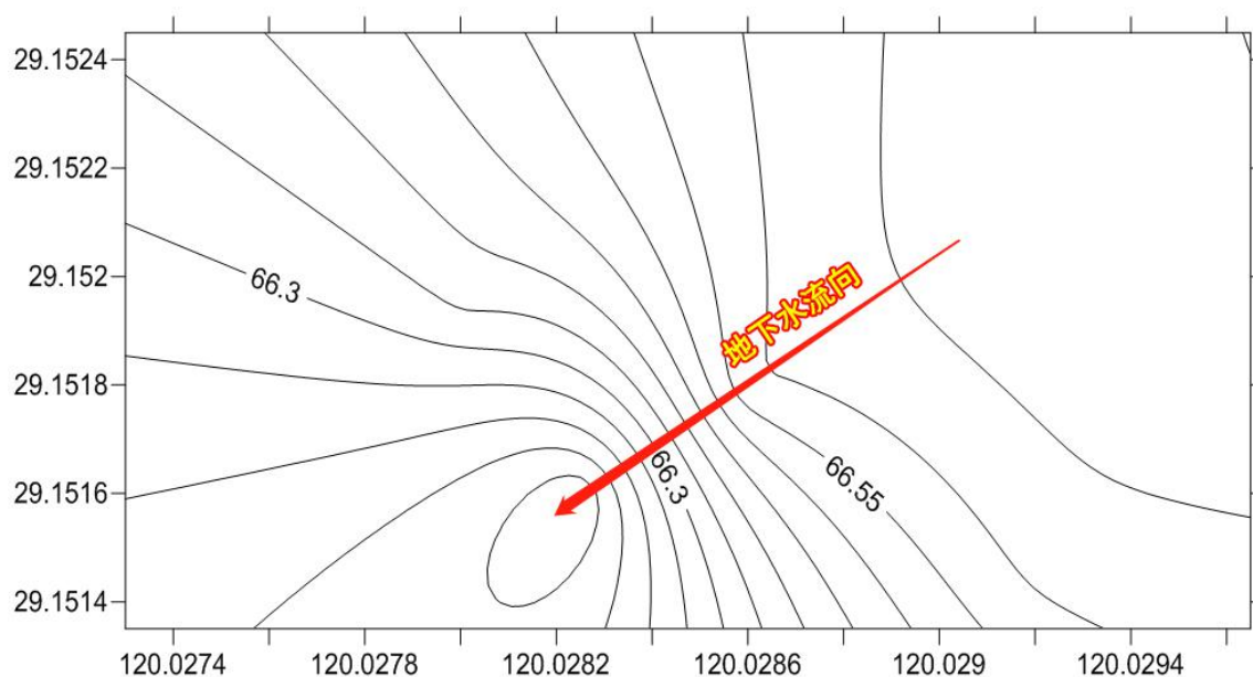
图 2.5-2 地下水流向等值线图
