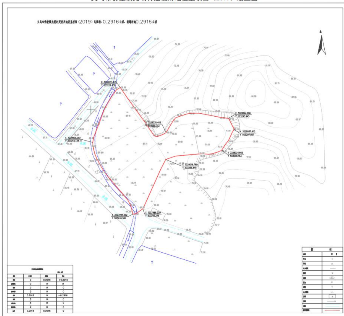
义乌市佛堂镇光明村建设用地复垦项目（2019）竣工图
